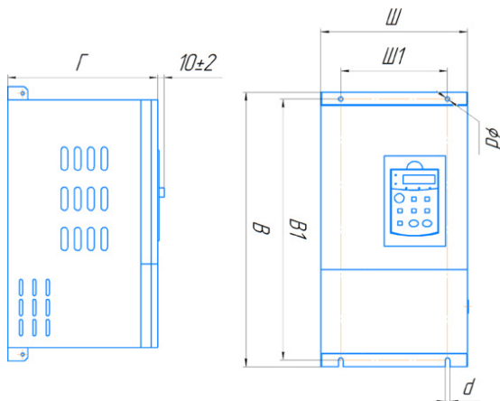
Рис. 2.5.26 Габаритные и установочные размеры устройств серии LCI в металлическом корпусе
